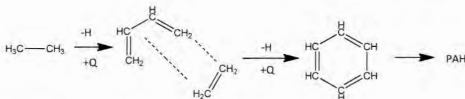
Σχήμα 4.5. Πυροσύνθεση PAH από αιθάνιο
