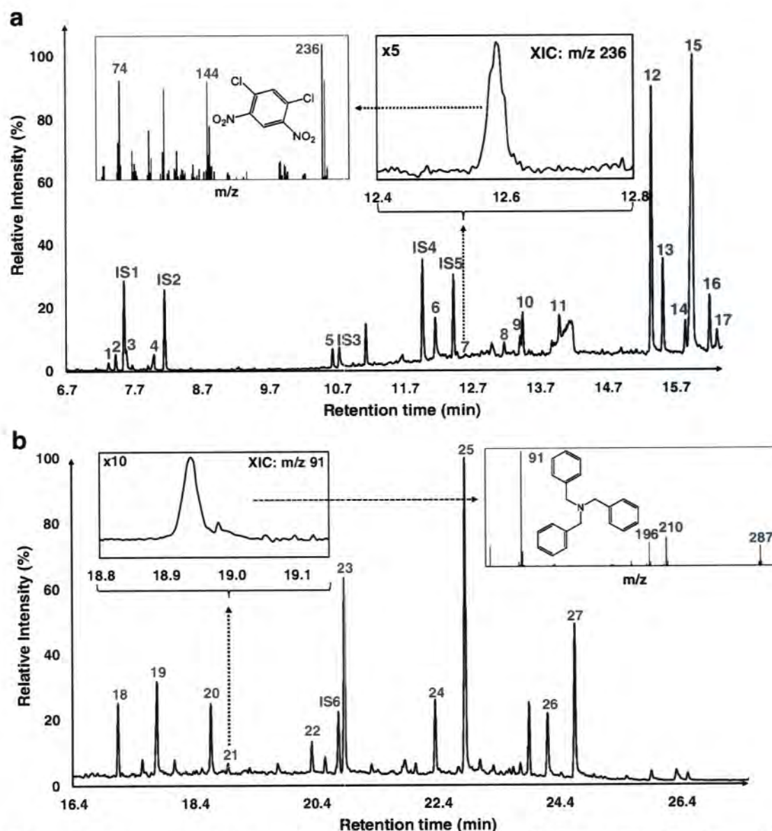
Σχήμα 5.1. Χρωματογράφημα πολυεστερικού υφάσματος αθλητικού μπουφάν. IS1 – IS6: εσωτερικά πρότυπα.
