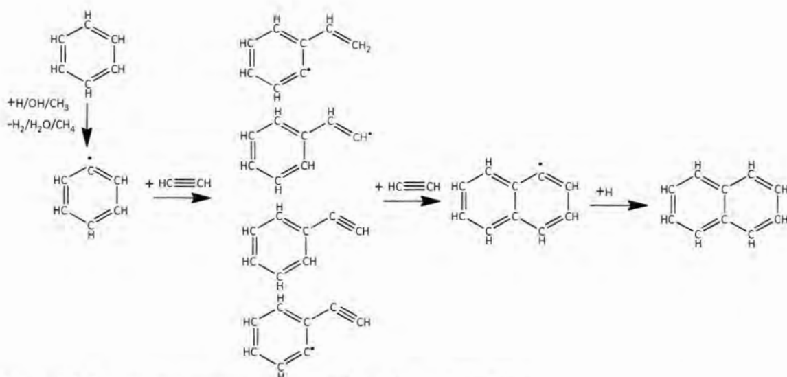
Σχήμα 4.6. Μηχανισμός σχηματισμού ναφθαλενίου από βενζόλιο
