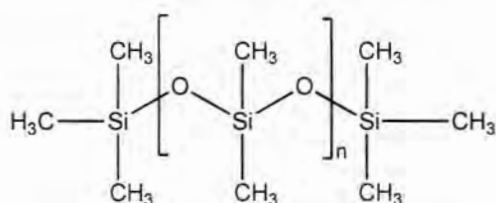
Σχήμα 3.1. Χημικός τύπος πολυδιμεθυλοσιλοξανίου
